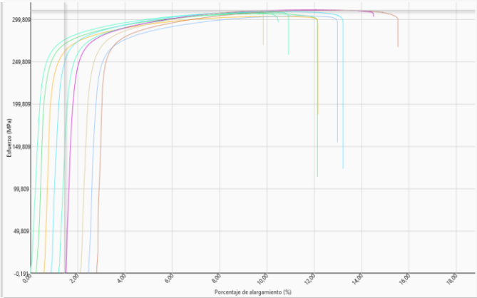
Grafica:Probeta plana
