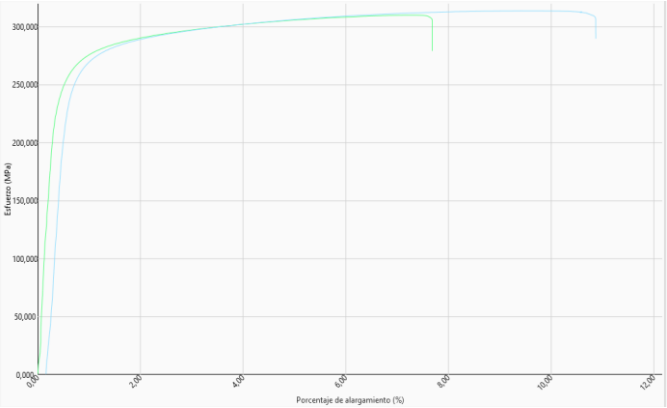
Grafica:Probetas planas
