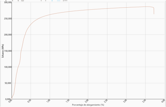
Grafica:Probetas cilindricas 6mm
