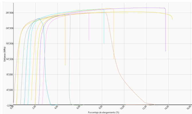
Grafica:Probetas planas
