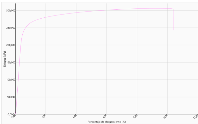
Grafica:Probetas cilindricas 6mm
