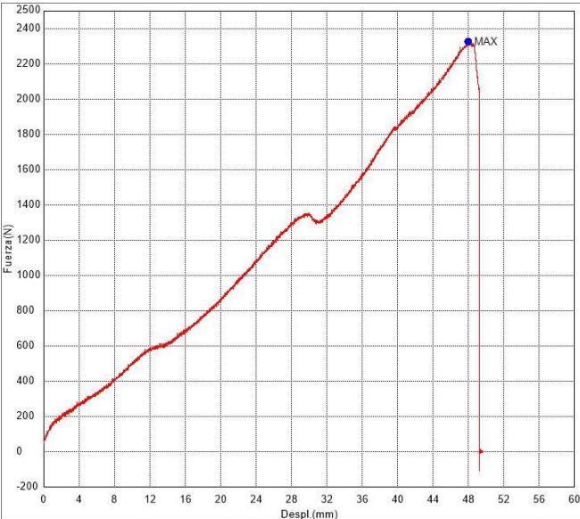
Gráfico de ensayo (Pieza 2)
