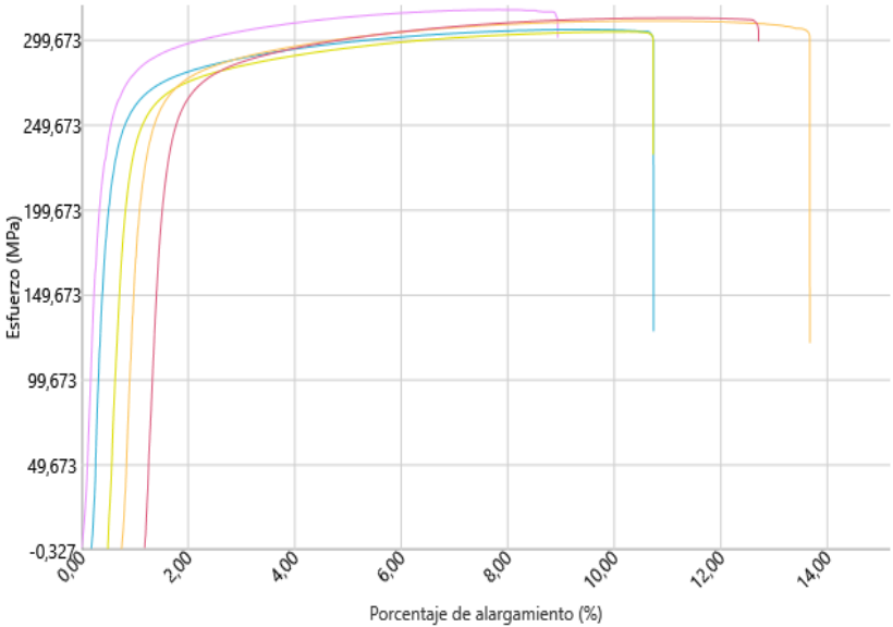
Gráfica de pruebas (Test chart)
