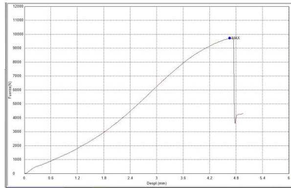
Grafica 1. Ejemplo de ensayo. Graph 1. Test example
