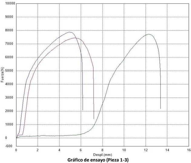
Gráfico de ensayo (Pieza 1-3)
