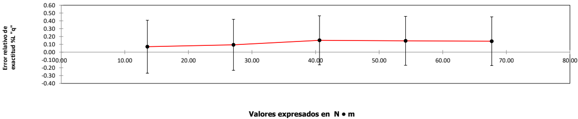
Gráfica del error relativo de exactitud (ANTIHORARIO)
