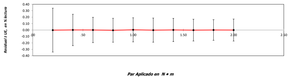
Gráfica de Residual de la Ecuación de mejor ajuste e incertidumbre Vs Par Aplicada (Antihorario)
