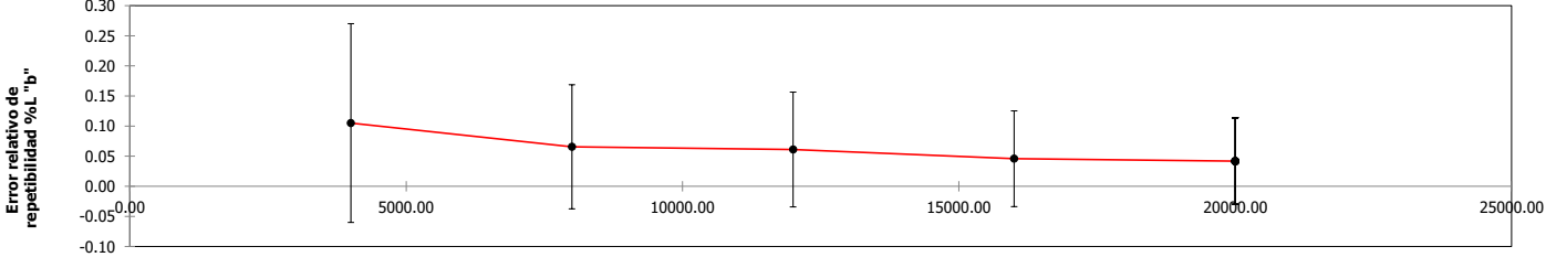
Gráfica del error relativo de repetibilidad (Tracción) (Graph of relative repeatability error (Traction))
