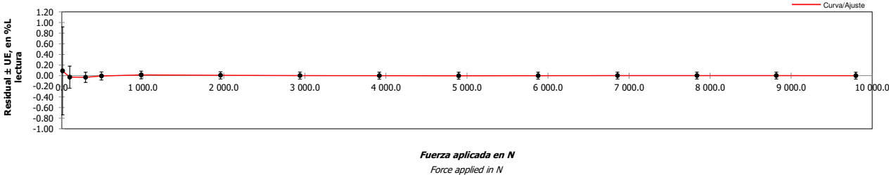
Gráfica de residual de la ecuación de mejor ajuste e incertidumbre Vs Fuerza aplicada (Tracción) (Residual graph of the best fit and uncertainty equation Vs Applied force (Traction))
