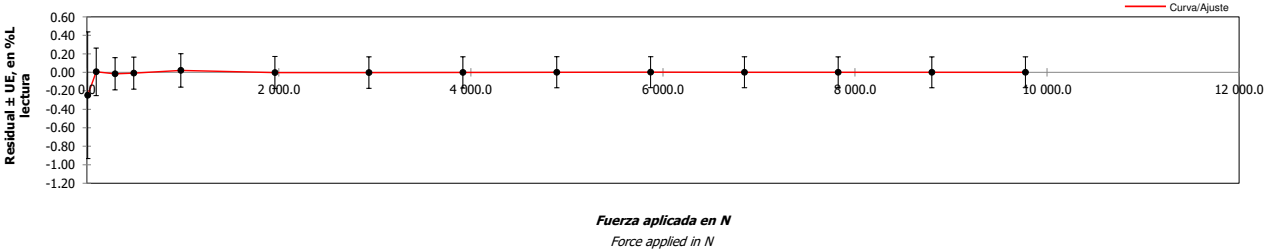
Gráfica de residual de la ecuación de mejor ajuste e incertidumbre Vs Fuerza aplicada (Compresión) (Residual graph of the best fit and uncertainty equation Vs Applied force (Compression))
