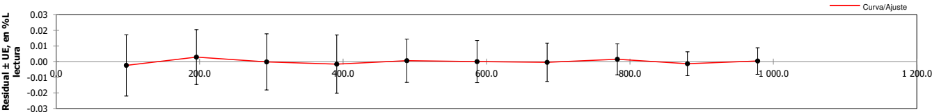
Gráfica de residual de la ecuación de mejor ajuste e incertidumbre Vs fuerza aplicada (Compresión) (Residual graph of the best fit and uncertainty equation Vs applied force (Compression))
