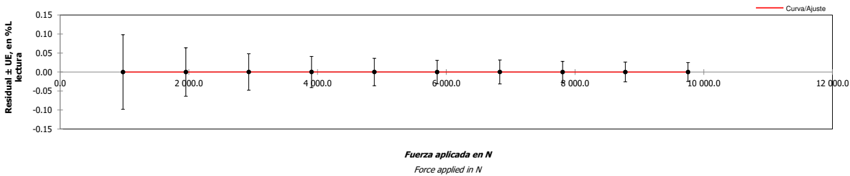
Gráfica de residual de la ecuación de mejor ajuste e incertidumbre Vs Fuerza aplicada (Tracción) (Residual graph of the best fit and uncertainty equation Vs Applied force (Traction))
