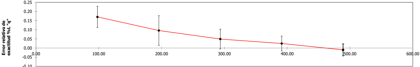
Gráfica del error relativo de exactitud (Tracción) (Graph of relative accuracy error (Traction))
