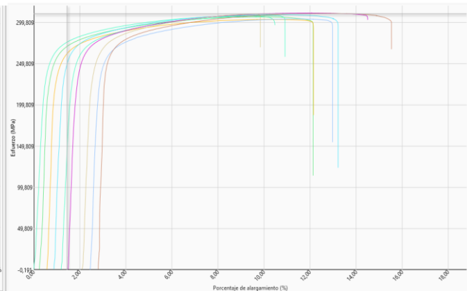
Grafica: Probeta plana
