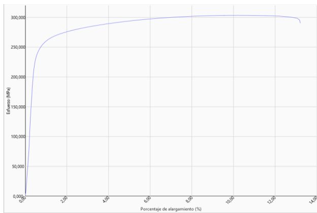
Grafica: Probeta cilíndrica 6 mm
