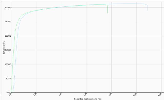
Grafica:Probetas planas
