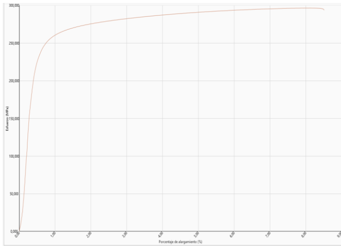
Gráfico 2. Items, diametro Ø 6 mm.
