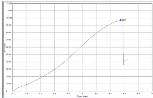
Gráfica 1. Ejemplo de ensayo. Graph 1. Test example
