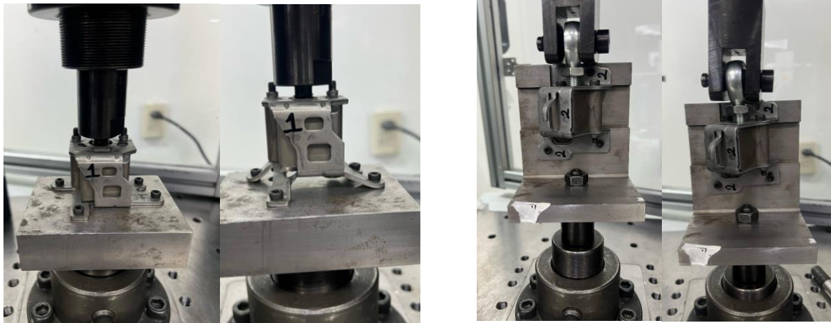
Imagen 2. Ensayo.
