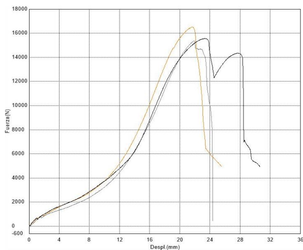
Gráfico de ensayo (Pieza 1-3)
