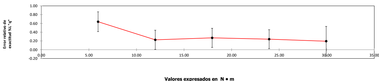
Gráfica del error relativo de exactitud (HORARIO)
