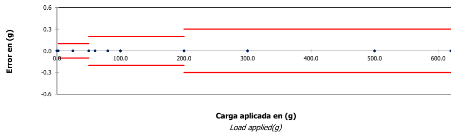
Grafica de errores de indicación Chart for errors of indication
