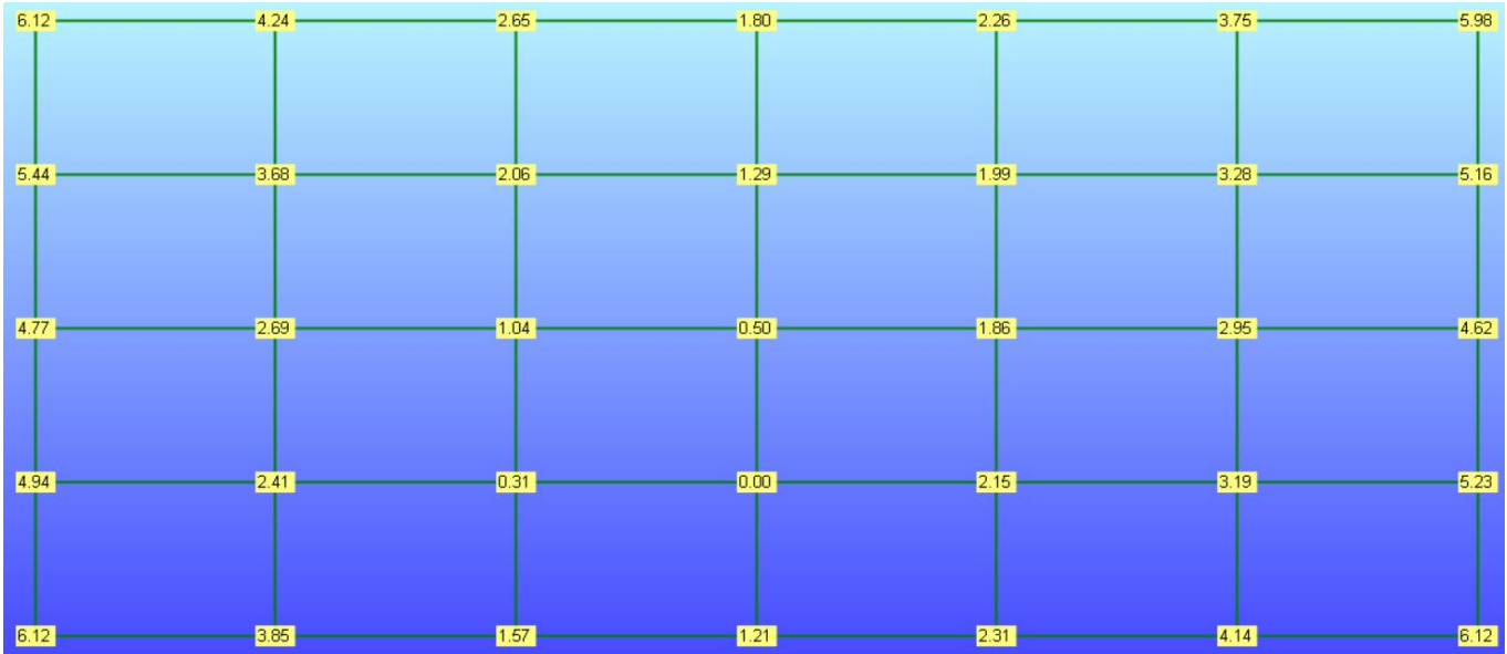
Desviaciones encontradas en toda la superficie de medición de la mesa de planitud (Deviations found over the entire measurement surface of the flatness table)
