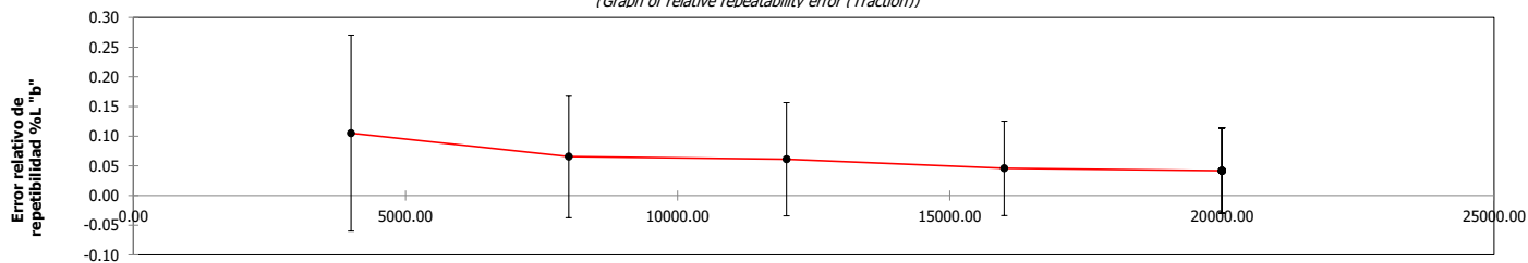
Gráfica del error relativo de repetibilidad (Tracción) (Graph of relative repeatability error (Traction))
