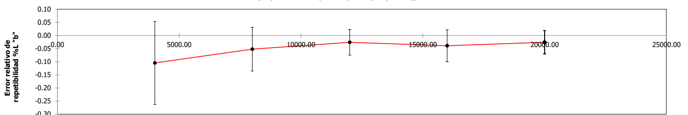
Gráfica del error relativo de repetibilidad (Compresión) (Graph of relative repeatability error (Compression))
