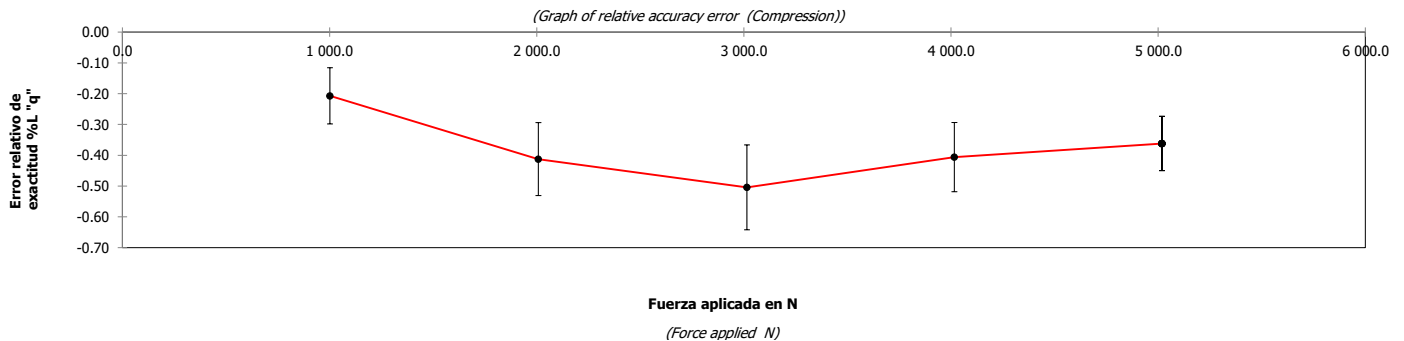
Gráfica del error relativo de exactitud (Compresión)
