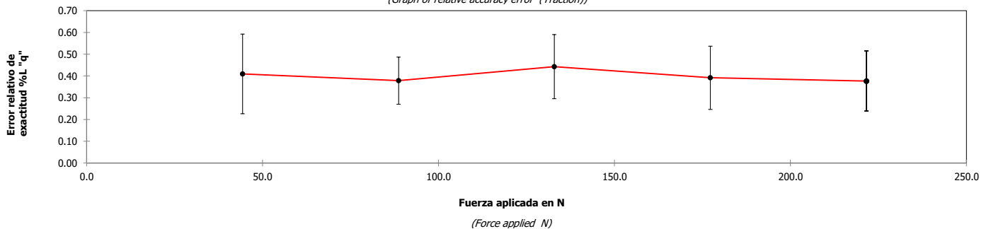
Gráfica del error relativo de exactitud (Tracción)
