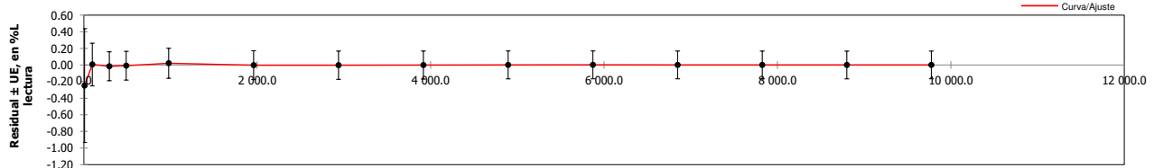
Gráfica de residual de la ecuación de mejor ajuste e incertidumbre Vs Fuerza aplicada (Compresión) (Residual graph of the best fit and uncertainty equation Vs Applied force (Compression))
