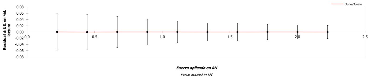
Gráfica de residual de la ecuación de mejor ajuste e incertidumbre Vs Fuerza aplicada (Compresión) (Residual graph of the best fit and uncertainty equation Vs Applied force (Compression))
