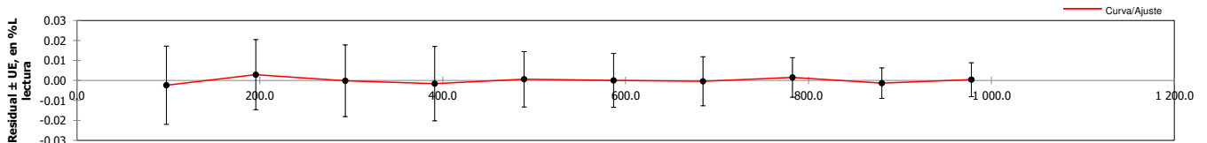
Gráfica de residual de la ecuación de mejor ajuste e incertidumbre Vs fuerza aplicada (Compresión) (Residual graph of the best fit and uncertainty equation Vs applied force (Compression))
